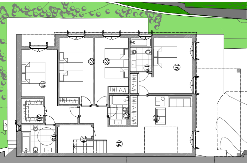
PLANTA DO PISO -1
